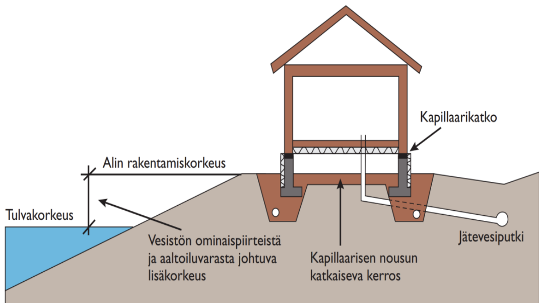
Kuva 2 Alin suositeltava rakentamiskorkeus tuulettuvalle alapohjalle. Lähde Ympäristöopas 2014
